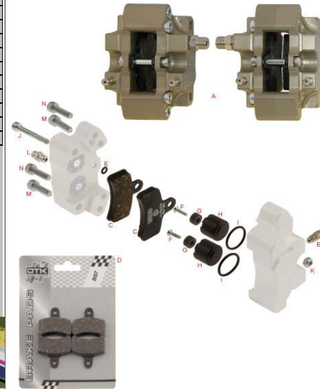
Tav. 35 PINZA FRENO ANTERIORE • FRONT BRAKE CALIPER BS7
