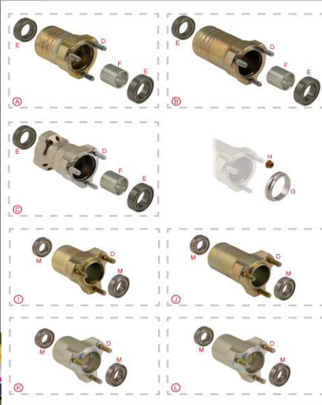
Tav. 17 MOZZI RUOTA ANTERIORI • FRONT WHEELS HUBS
